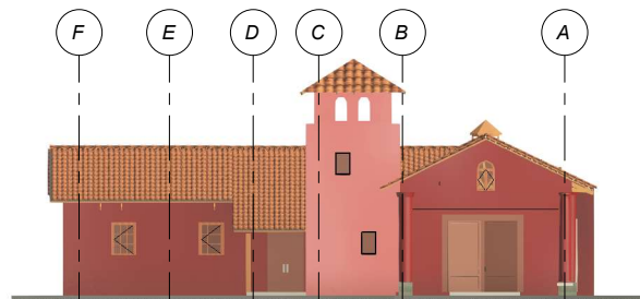
3 Este A101 1:150
