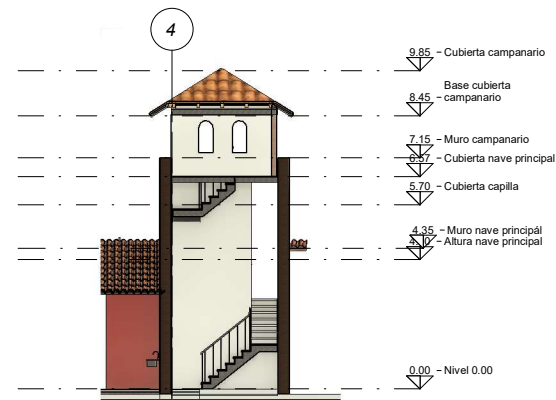
4 Sección 4 A101 1:100
